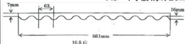
スレート小波(厚み20mm)
