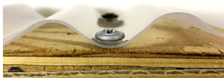
谷打ち詳細図
